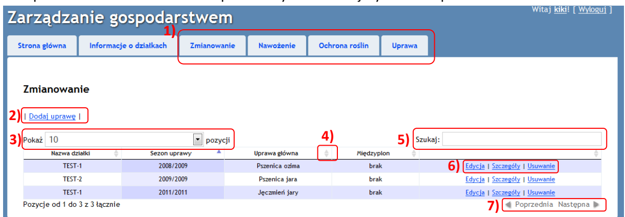
Rysunek 1. Przykładowe okno programu.
